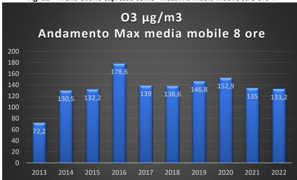
Fig. 22 – Trend Ozono espresso come “Massima media mobile su 8 ore”.
