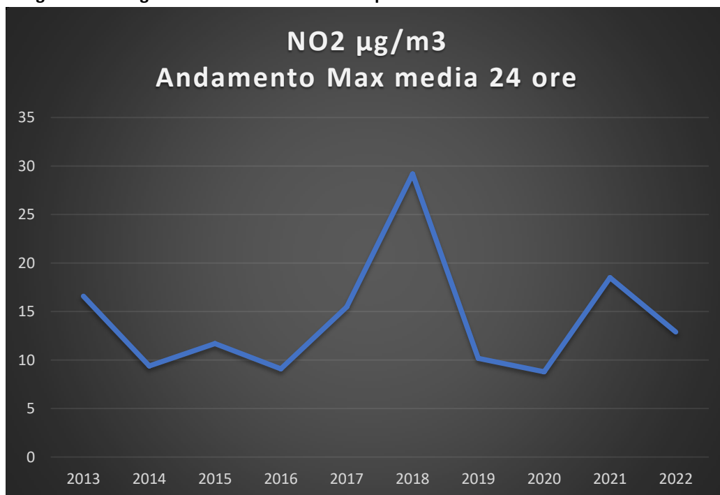
Fig. 21 – Trend grafico del Biossido d’Azoto espresso come “Massimo valore sulle 24 ore”
