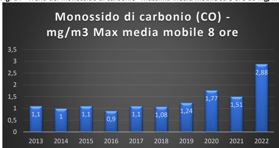
Fig. 14 - Trend del monossido di carbonio "Massima media mobile su 8 ore 10 mg/m 3 "
