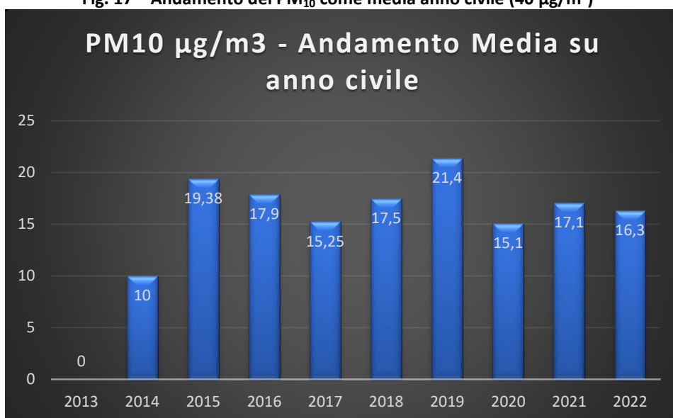
Fig. 17 – Andamento del PM 10 come media anno civile (40 µg/m 3 )”
