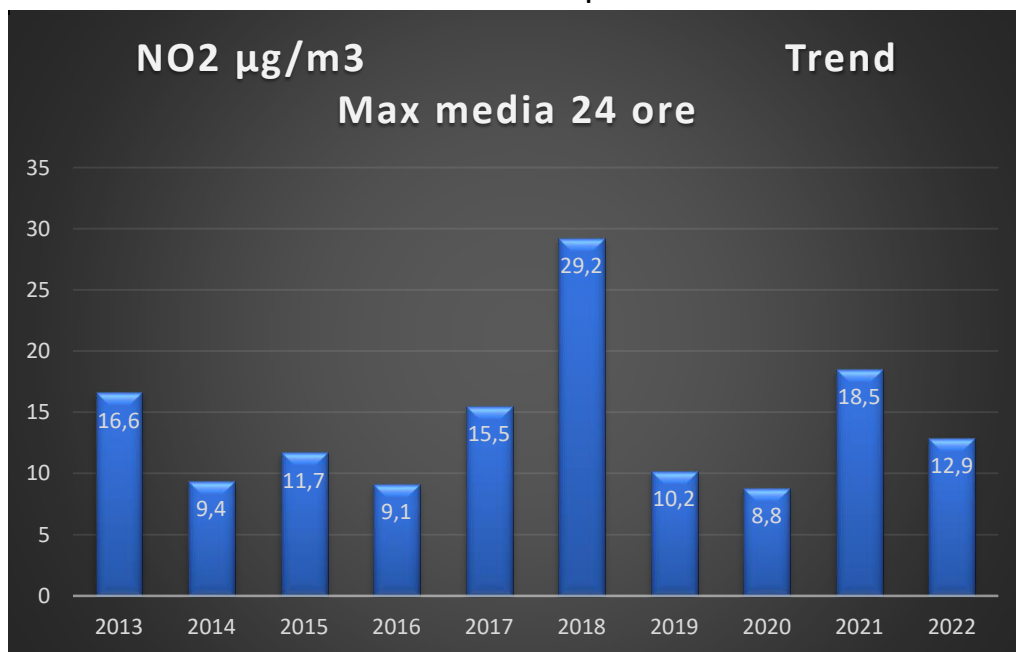
Fig. 20 – Tendenza delle concentrazioni del Biossido d’Azoto espresso come “Massimo valore medio sulle 24 ore”
