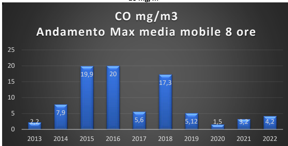
Fig. 25 - Trend del monossido di carbonio "Massima media mobile su 8 ore 10 mg/m 3 "
