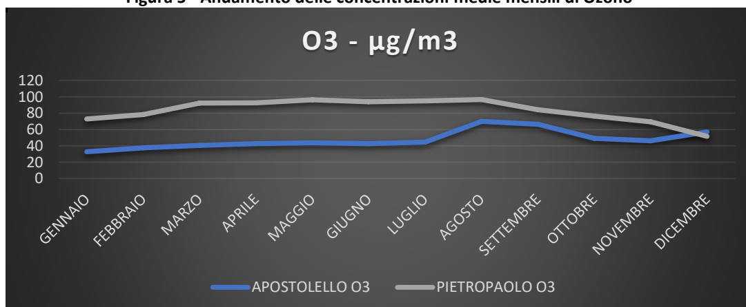
Figura 5 - Andamento delle concentrazioni medie mensili di Ozono
