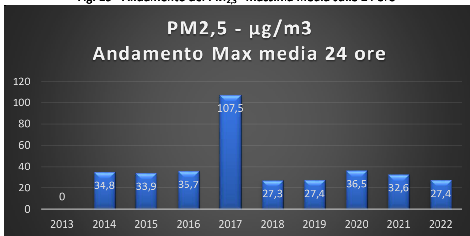
Fig. 29 - Andamento del PM 2,5 “Massima media sulle 24 ore”
