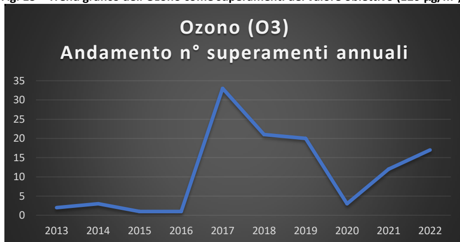
Fig. 13 – Trend grafico dell’Ozono come superamenti del valore obiettivo (120 µg/m 3 )”
