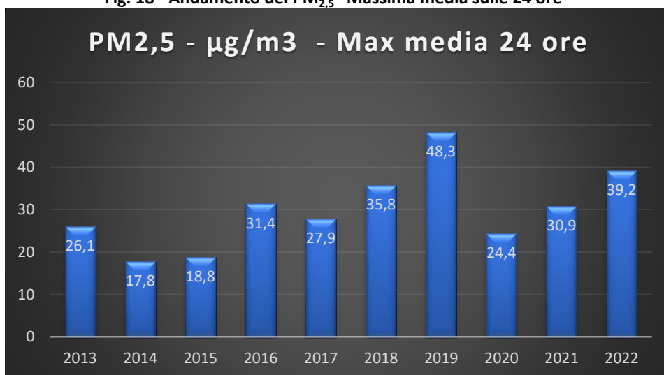
Fig. 18 - Andamento del PM 2,5 “Massima media sulle 24 ore”
