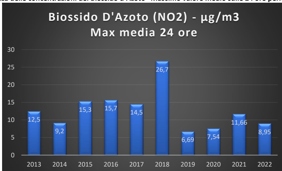
Fig. 9 – Tendenza delle concentrazioni del Biossido d'Azoto "Massimo valore medio sulle 24 ore periodo 2013 – 2022
