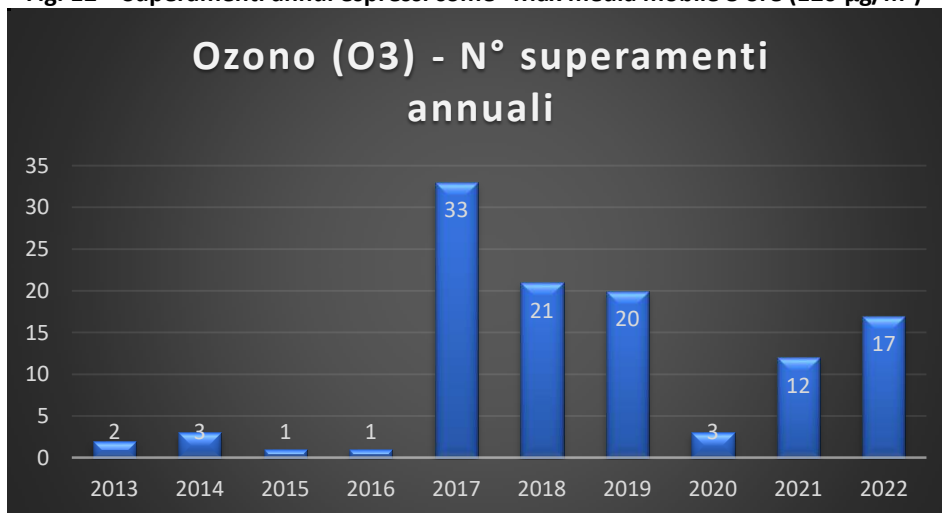
Fig. 12 – Superamenti annui espressi come “Max media mobile 8 ore (120 µg/m 3 )”
