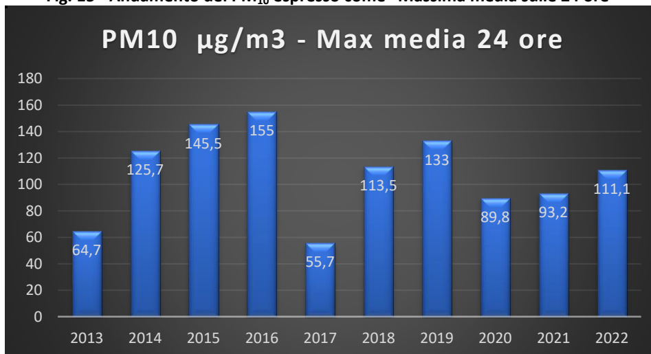
Fig. 15 - Andamento del PM 10 espresso come "Massima media sulle 24 ore"
