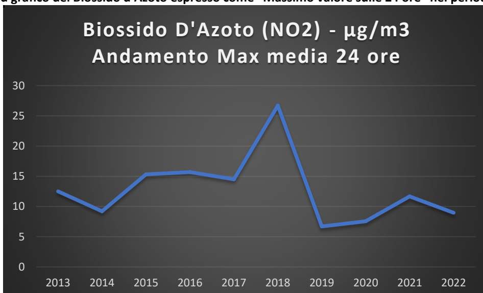
Fig. 10 – Trend grafico del Biossido d'Azoto espresso come "Massimo valore sulle 24 ore" nel periodo 2013 – 2022
