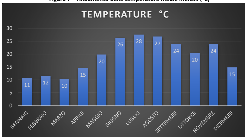
Figura 7 – Andamento delle temperature medie mensili (°C)
