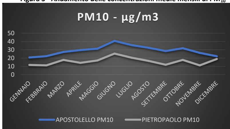
Figura 3 - Andamento delle concentrazioni medie mensili di \text{PM}_{10}
