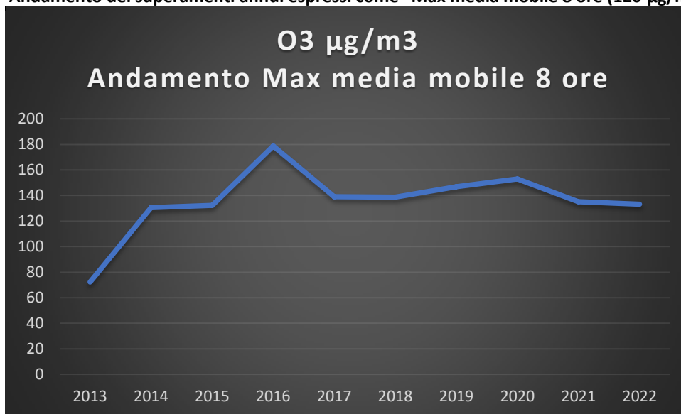
Fig. 24 – Trend grafico dell’Ozono come superamenti del valore obiettivo (120 µg/m 3 )”
