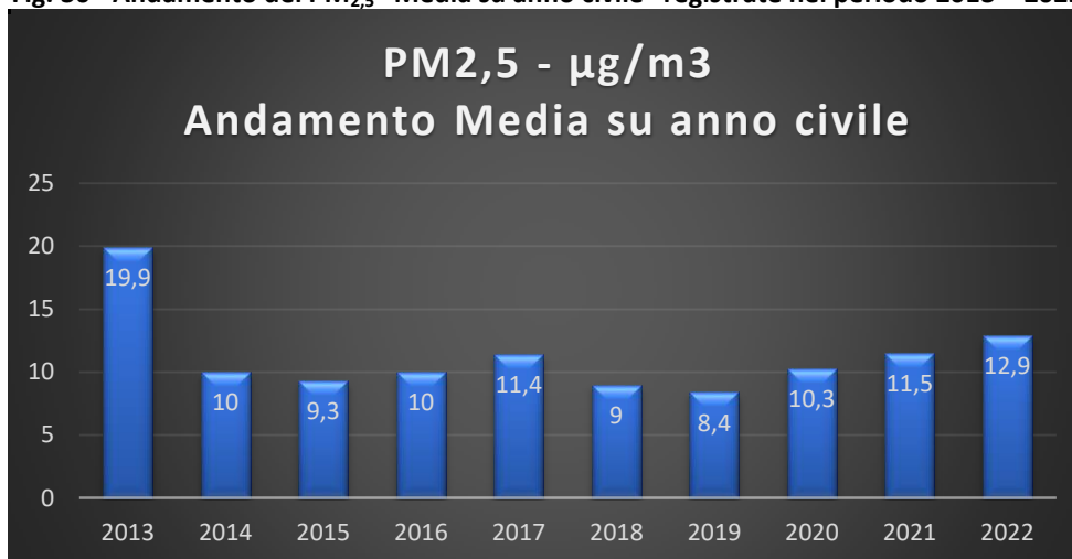
Fig. 30 - Andamento del PM 2,5 “Media su anno civile” registrate nel periodo 2013 – 2022
