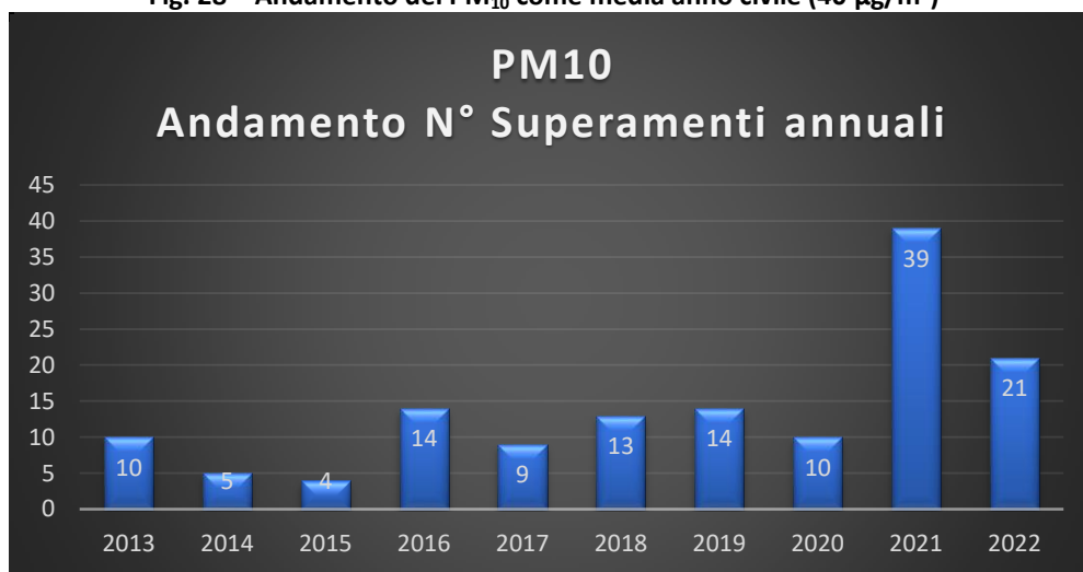
Trend PM 2,5 periodo 2013-2022
