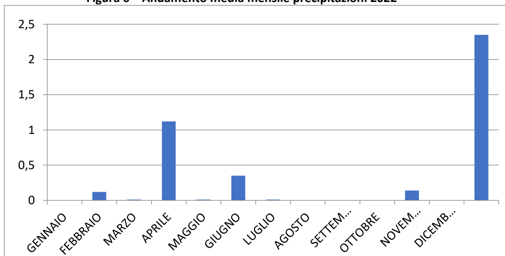
Figura 6 – Andamento media mensile precipitazioni 2022 –
