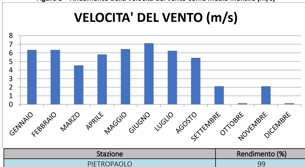
Figura 8 – Andamento della velocità del vento come media mensile (m/s)
