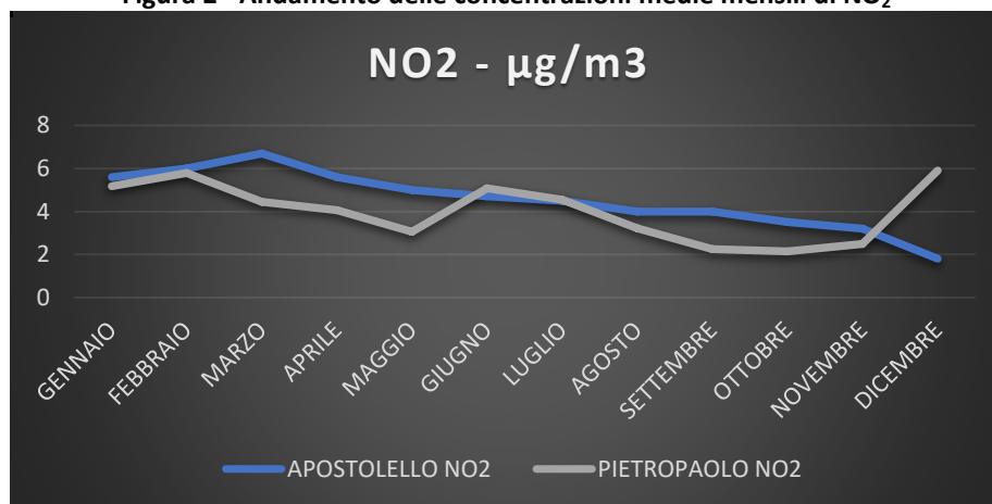
Figura 2 - Andamento delle concentrazioni medie mensili di NO 2
