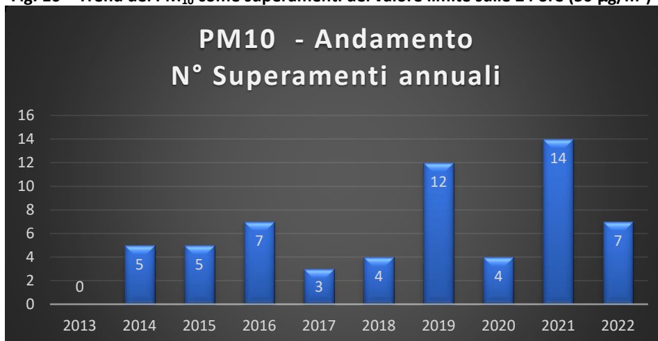
Fig. 16 – Trend del PM 10 come superamenti del valore limite sulle 24 ore (50 µg/m 3 )
