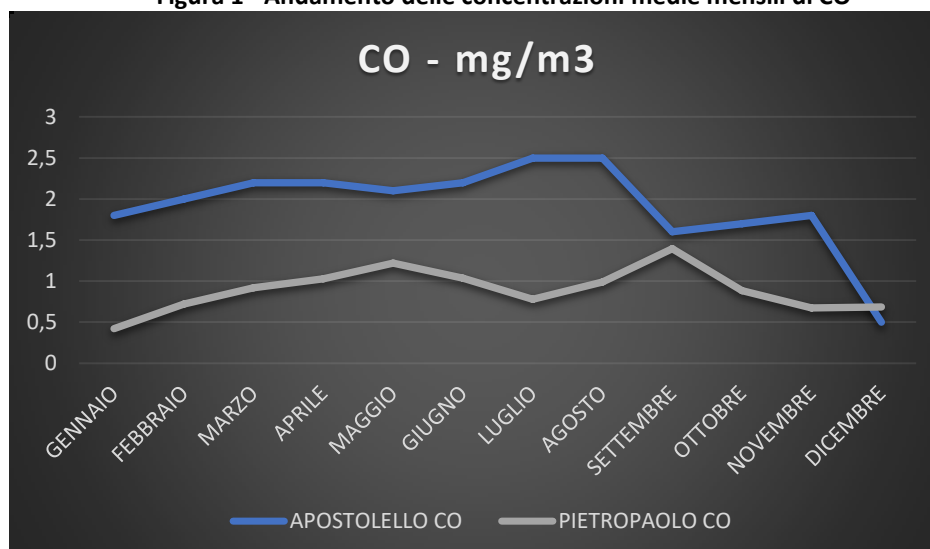
Figura 1 - Andamento delle concentrazioni medie mensili di CO
