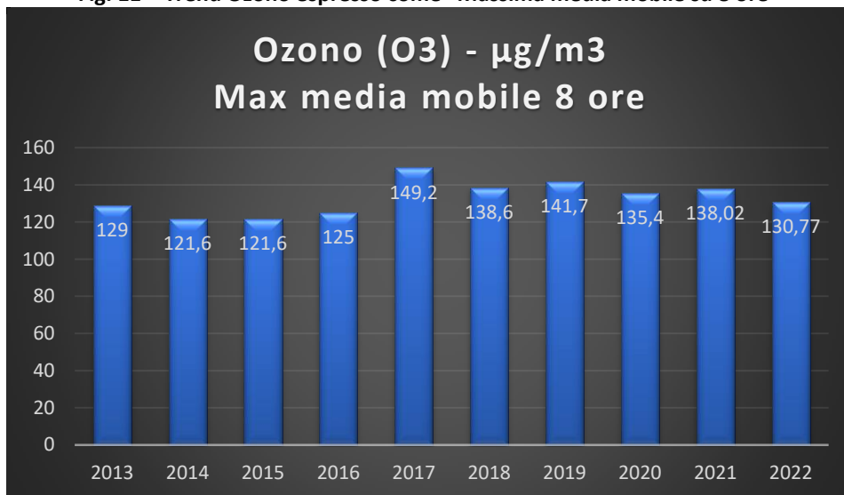
Fig. 11 – Trend Ozono espresso come “Massima media mobile su 8 ore”
