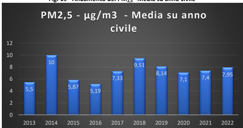
Fig. 19 - Andamento del PM 2,5 “Media su anno civile”
