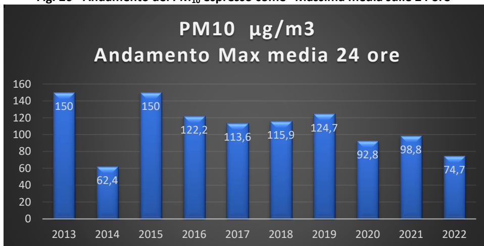
Fig. 26 - Andamento del PM 10 espresso come "Massima media sulle 24 ore"
