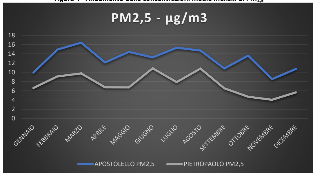
Figura 4 - Andamento delle concentrazioni medie mensili di PM 2,5
